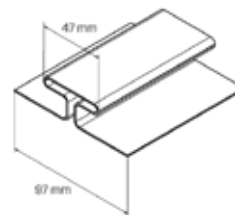
Montážna lišta H
